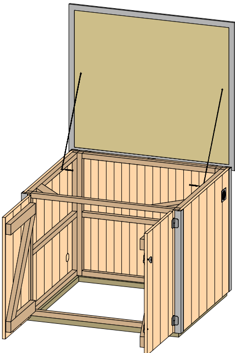
12 - Fixer le toit sur le fond avec les trois charnières (3 x 3 vis 5x50)
