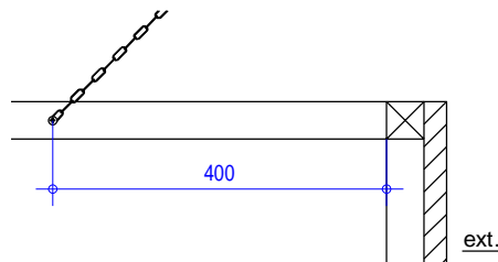
12 - Fixer le toit sur le fond avec les trois charnières (3 x 3 vis 5x50)
