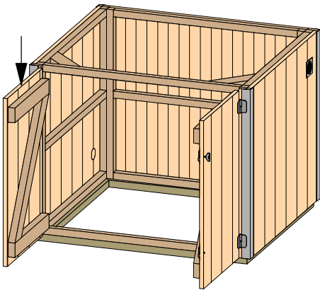
11 - Positionner la porte gauche avec les deux paumelles
