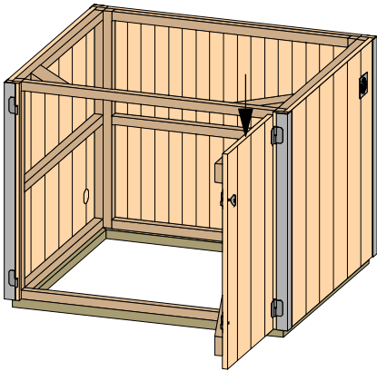
10 - Positionner la porte droite avec les deux paumelles
