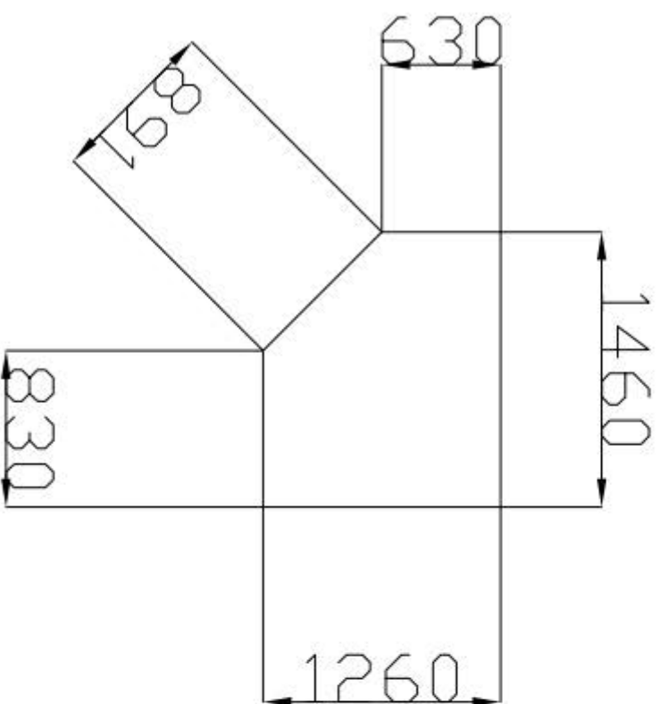
plan local cote extérieur
