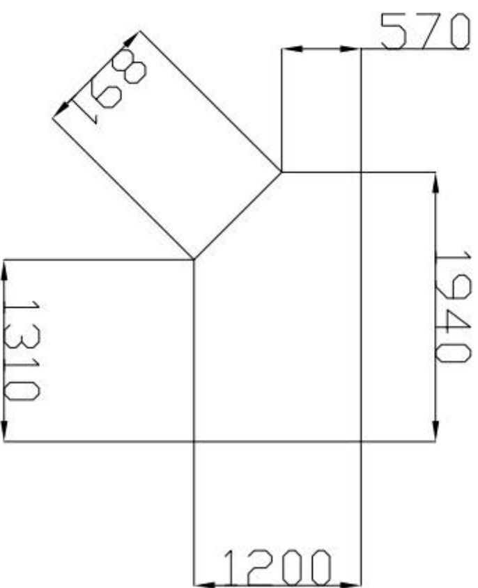
plan dalle
